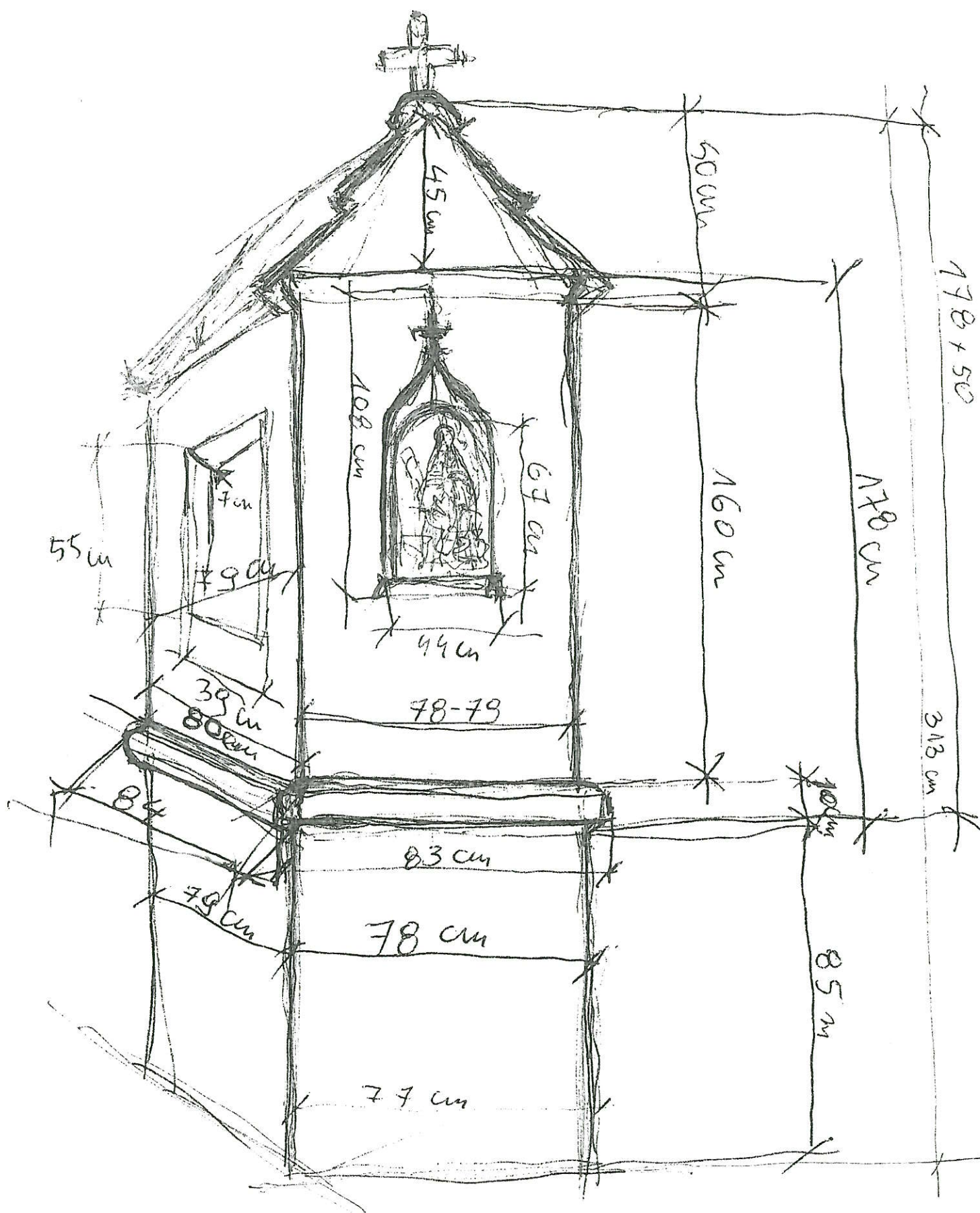
SZKICOWY, ROBOCZY OBMAR KAPLICZKI PRZY UL. FATIMSKIEJ 5 W KRAKOWIE
